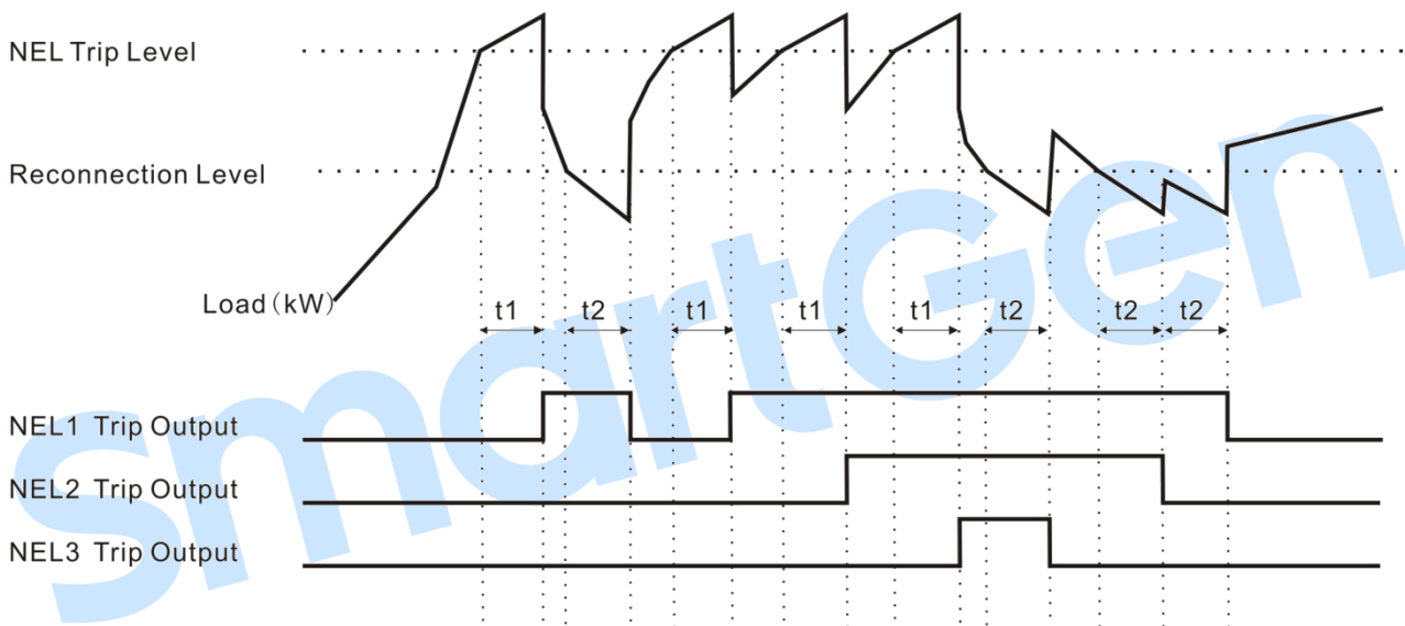
Fig. 10 – NEL Control Time Sequence
